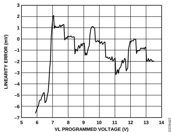
Figure 27. HVOOUT VHH Linearity Error
