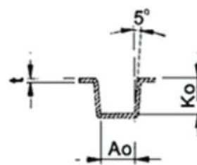
SEC: A-A'
