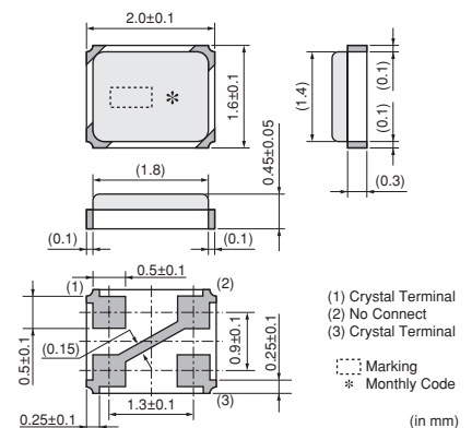
XRCPB_F_L/M 24.0000–48.0000MHz XRCPB_F_P 24.0000–32.0000MHz
