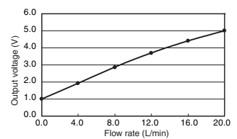
D6F-20A5-000
