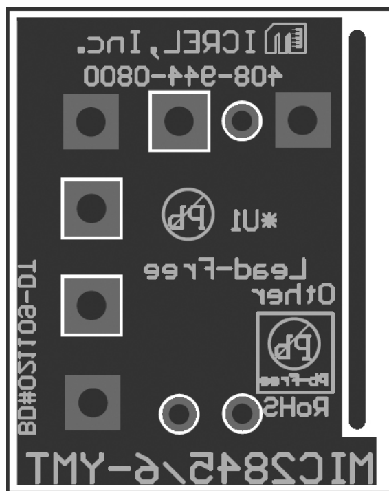
Bottom Layer
