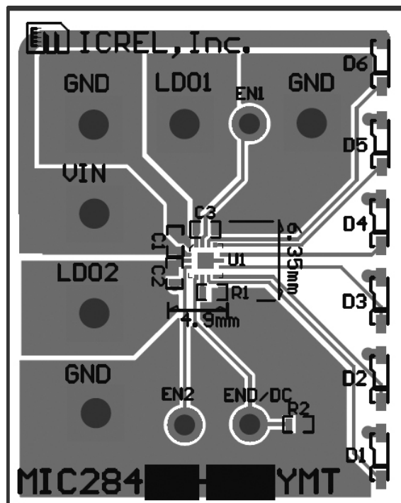
Top Layer
