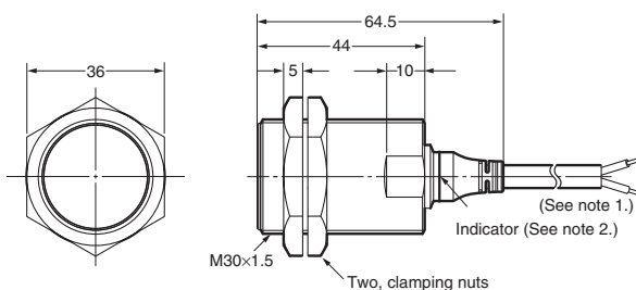
E2A-M30KS15-WP-□□
