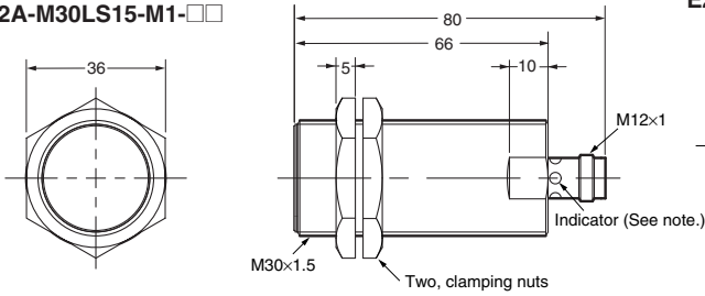
E2A-M30LS15-M1-□□
