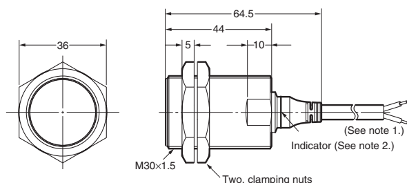
E2A-M30KS15-WP-□□
