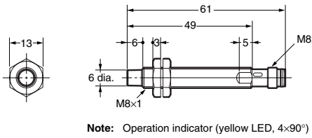
E2A-S08LN04-M5-□□
