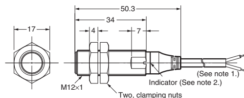
E2A-M12KS04-WP-□□
