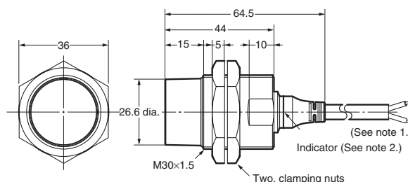
E2A-M30KN20-WP-□□
