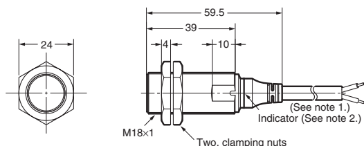
E2A-M18KS08-WP-□□
