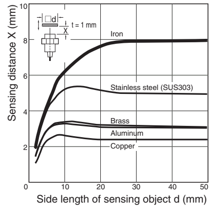
E2A-M12□N08
