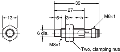
E2A-S08KN04-M5-□□
