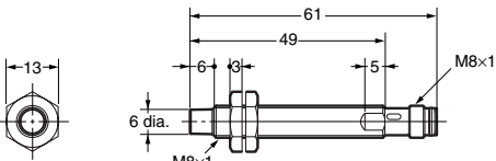
E2A-S08LN04-M5-□□
