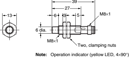
E2A-S08LN04-M5-□□
