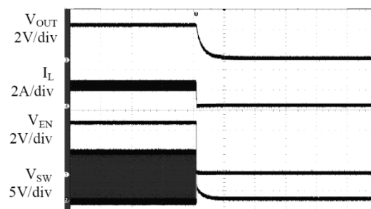
Fig. 13: Enable turn off ( R_{LOAD}=1.6\Omega )
