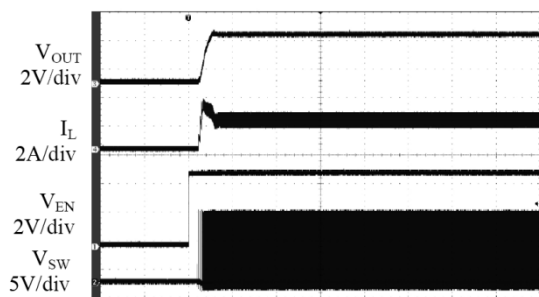
Fig. 12: Enable turn on ( R_{LOAD}=1.6\Omega )
