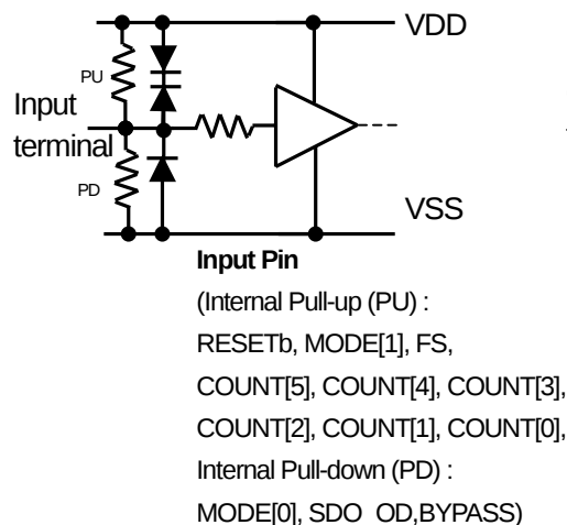
Fig. 3 I/O Equivalent Circuits
