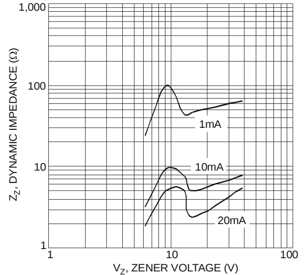
Fig. 4 Effect of Zener Voltage
