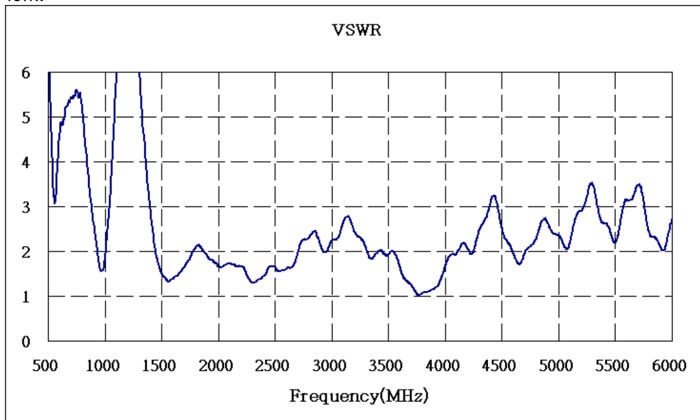
VSWR
