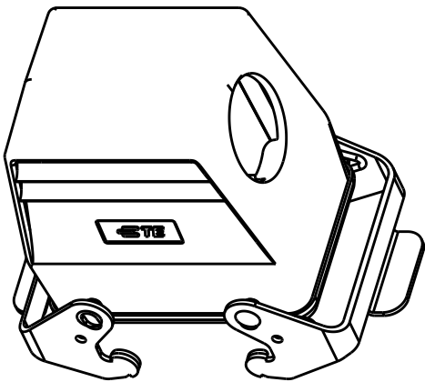
SCALE 1:2
