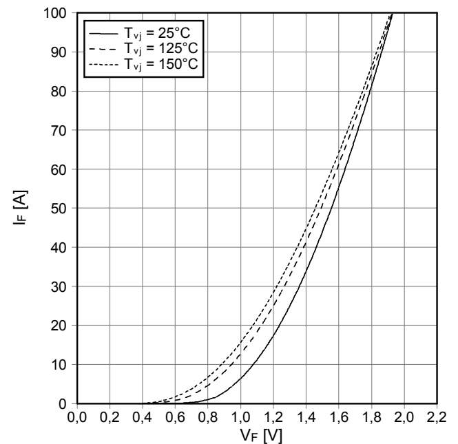
Durchlasskennlinie der Diode-Wechslr. (typisch) forward characteristic of diode-inverter (typical) I_F = f(V_F)
