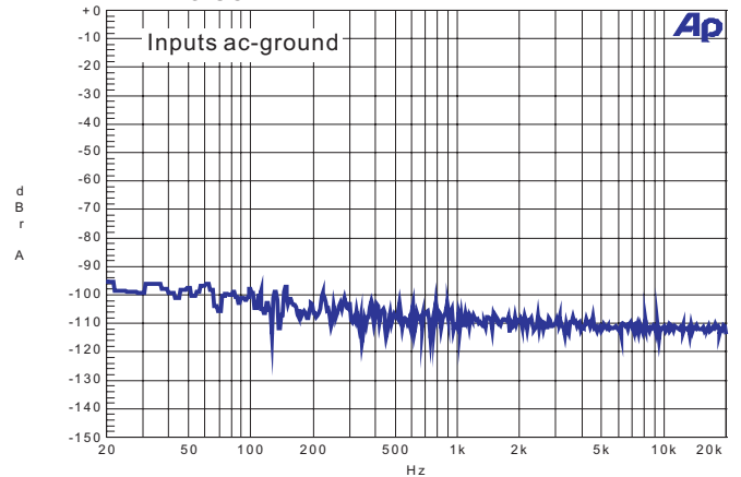
12. Noise FFT
