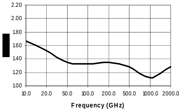
VSWR
