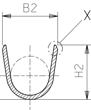
SECTION Z-Z SCHNITT Z-Z
