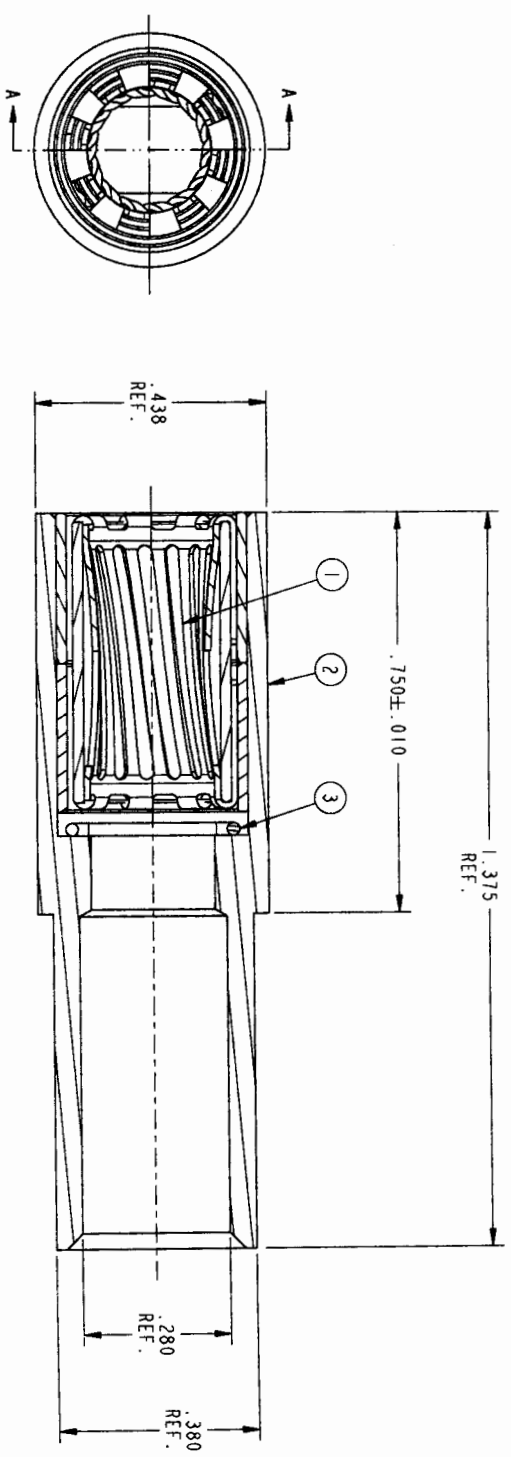
SECTION A-A
