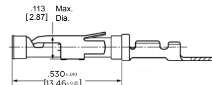
Socket
