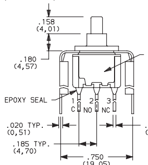
8121SD3_GE SPDT
