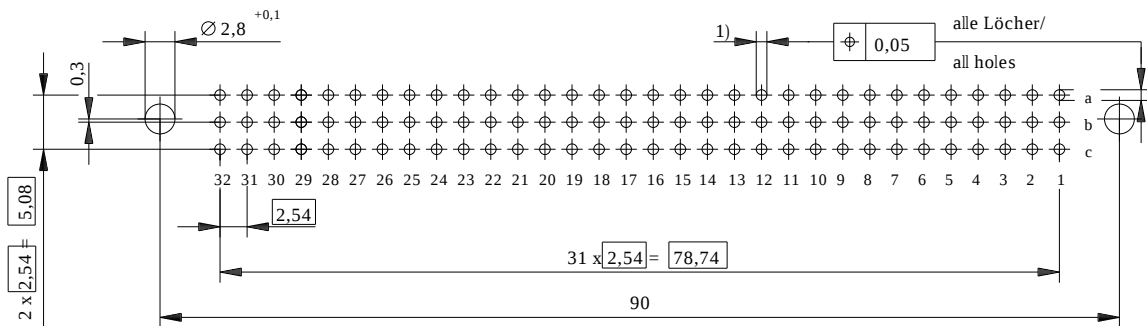
Leiterplatten-Lochbild /
