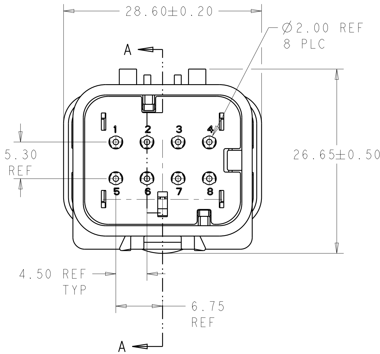
776538-1 SHOWN
