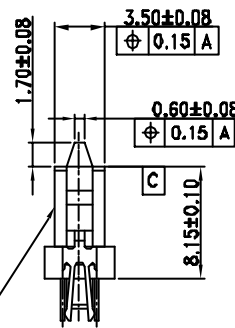
SECTION P-P 2:1
