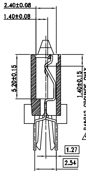
SECTION N-N 2:1
