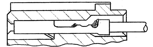
ファスチンファストン嵌合状態 (FASTIN-FASTON MATING STATE)
