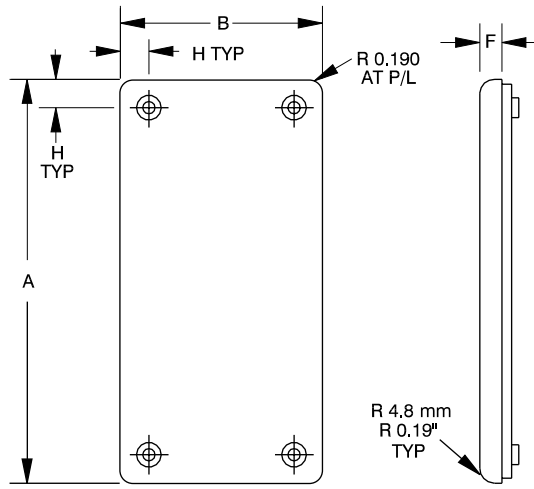
Lid View
