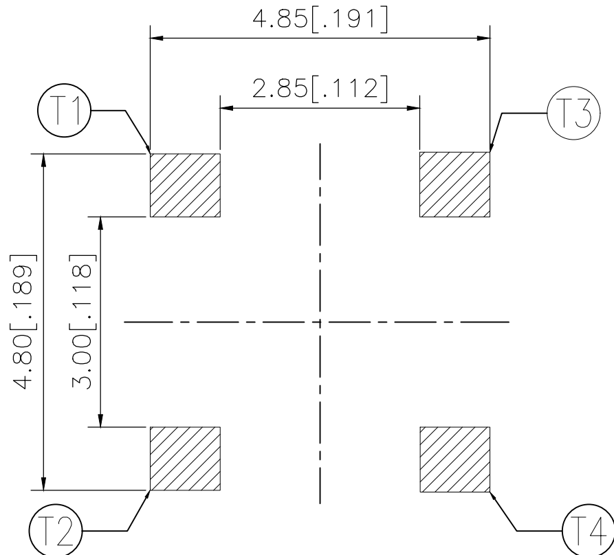
P.C.B. LAYOUT
