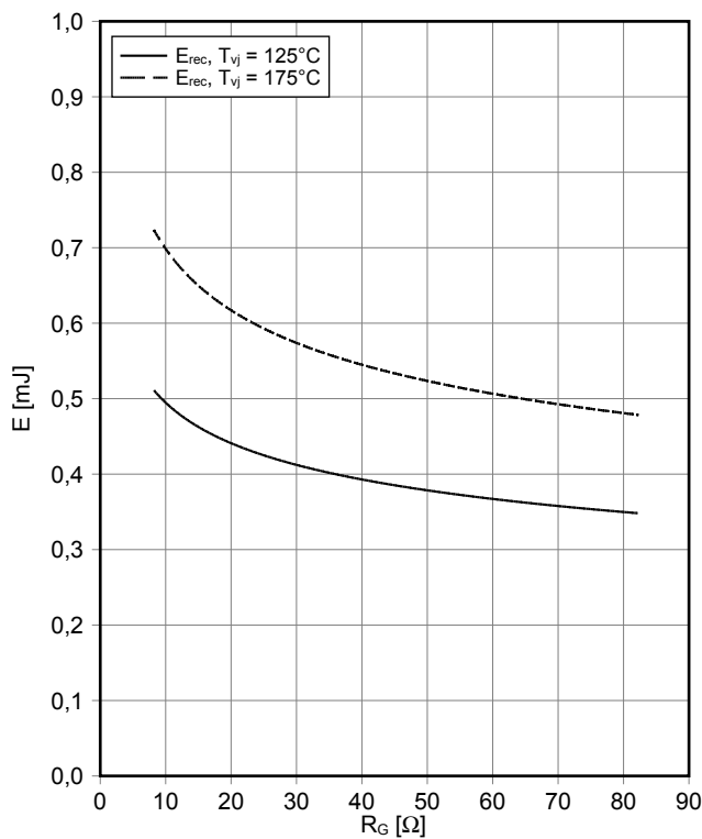
Schaltverluste Diode, Wechselrichter (typisch) switching losses Diode, Inverter (typical) E_{rec} = f(R_G) I_F = 10 \text{ A} , V_{CE} = 600 \text{ V}
