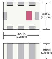
Case 41-2 (EIA 1210 / 3225)
