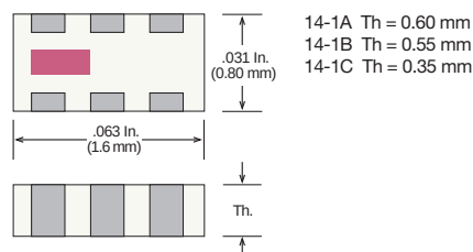
Case 14-1 (EIA 0603/ 1608)
