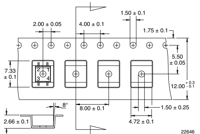
Fig. 13 - Tape Dimensions
