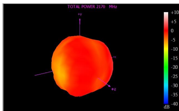
2170 MHz
