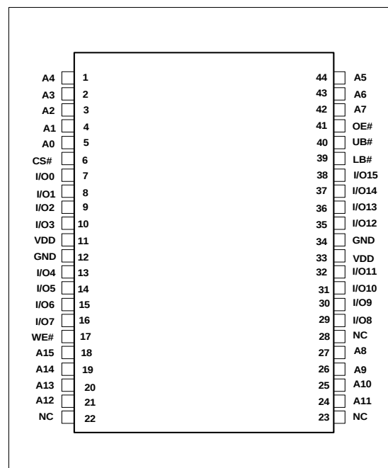
44-Pin mini TSOP (Type II)
