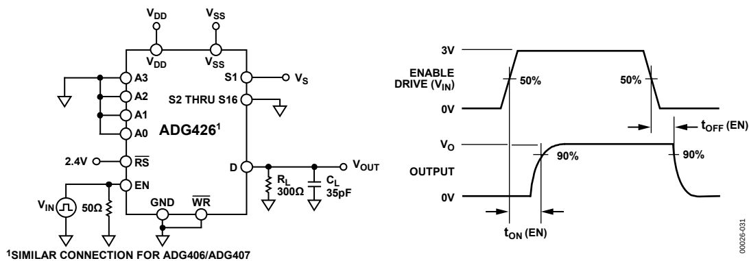
Figure 31. Enable Delay, t ON (EN), t OFF (EN)
