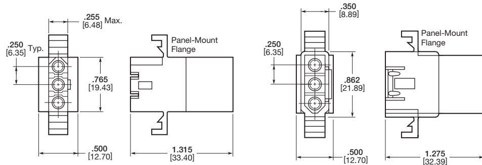
Receptacle
