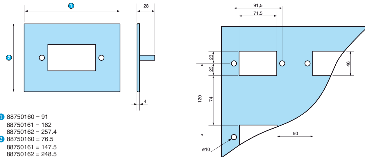
IP40
