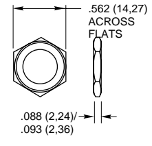
Hex Nut
