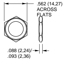
Hex Nut
