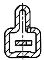
断面 "B"- "B" (SECT)
