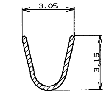
断面 "E"- "E" (SECT)
