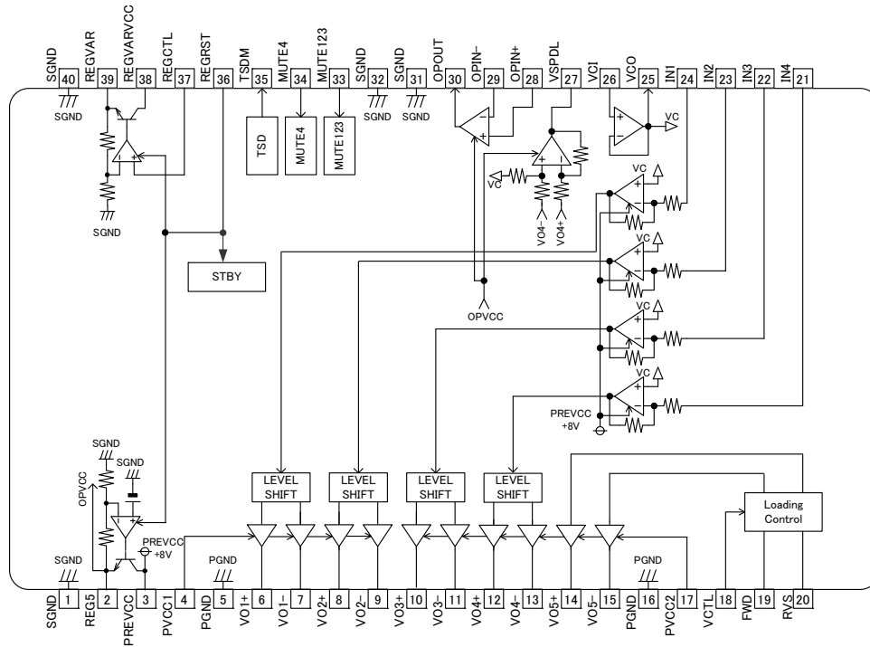
HTSSOP-B40
