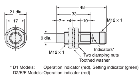
Diagram 23 E2E-X5MY□-M1
