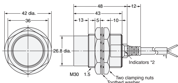
Diagram 17 E2E-X20MD□/E2E-X18ME□/F□ E2E-X18MY□
