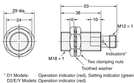
Diagram 26 E2E-X10D□-M1(G)/E2E-X10E□-M1/X10F□-M1 E2E-X10Y□-M1
