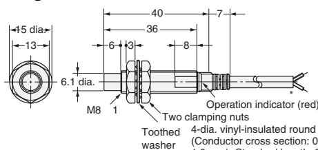
Diagram 8 E2E-X2MY□
