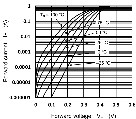
Fig. 9.1 I_F - V_F
