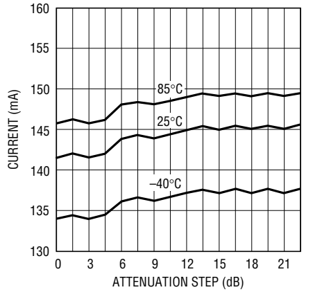
Total I_{\text{CC}} vs Attenuation Step
