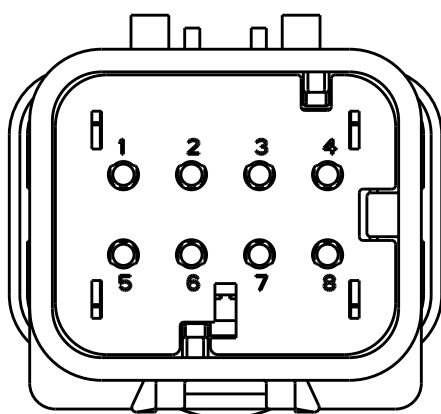
776495-4 SCALE 2:1
