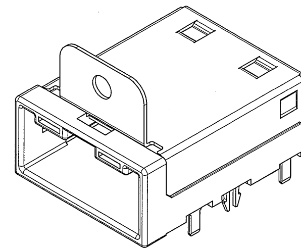
PERSPECTIVE VIEW (REF.) 斜視図 (参考)
