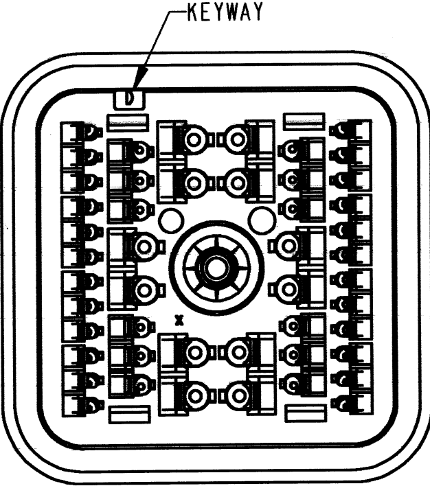
DRB16-48SDE-L018 KEY ARRANGEMENT -D-
