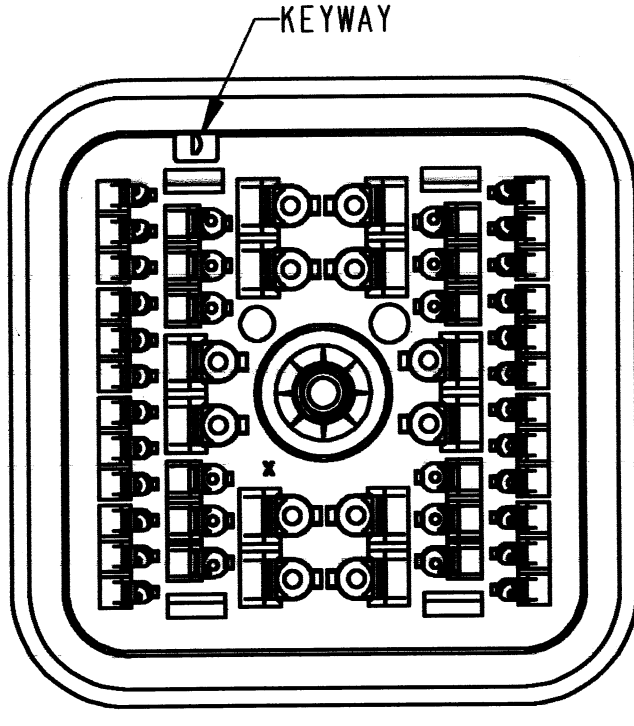
DRB16-48SDE-L018 KEY ARRANGEMENT -D-
