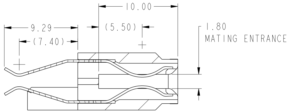
SECTION D-D
